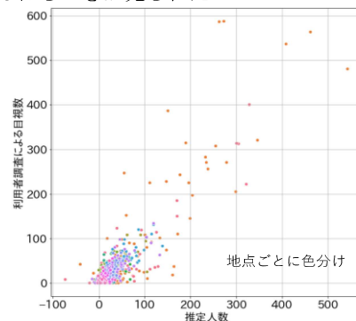
図 10 重回帰による推定人数と目視数
