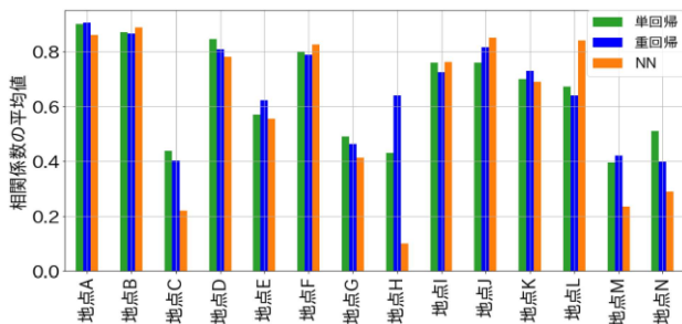
図 12 交差検定による相関係数の平均値
